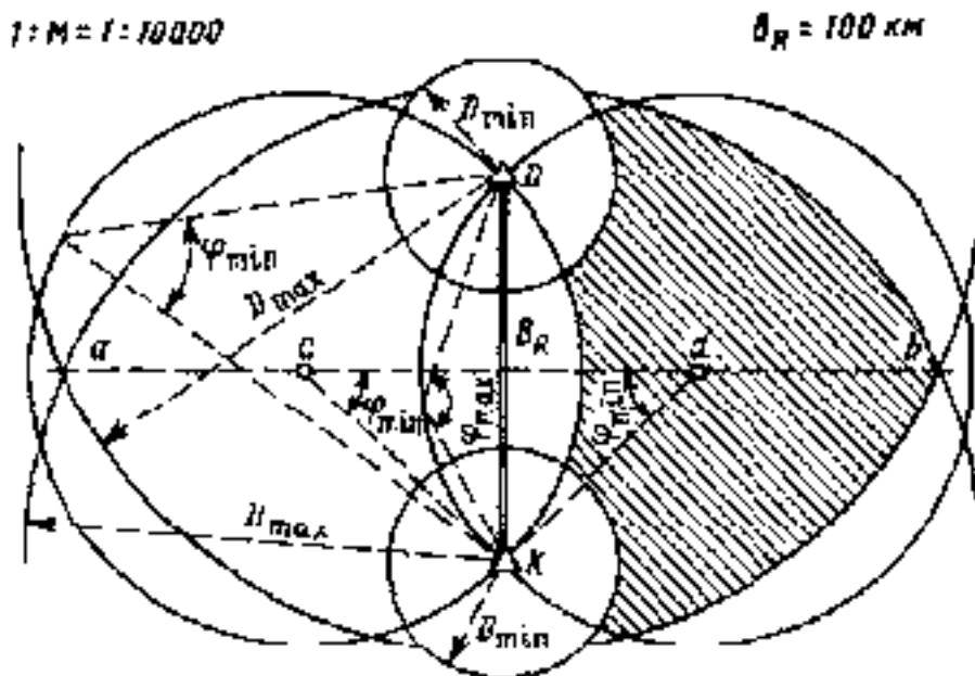
Рис. 39. Палетка рабочей зоны самолетного радиодальномера
