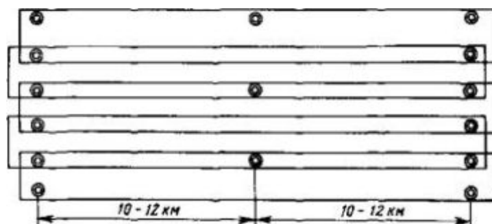
Рис. 5. Съемка в масштабе 1:10000 с сечением рельефа через 5,0 м
