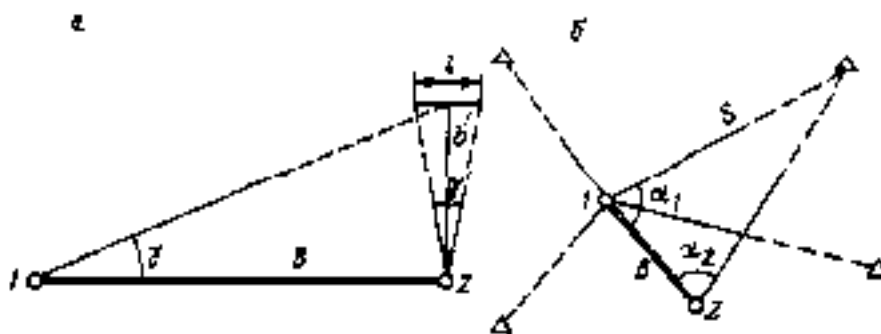
Рис. 37. Схемы определения длины базиса фотографирования: а) с помощью вспомогательного базиса; б) из неполного треугольника
