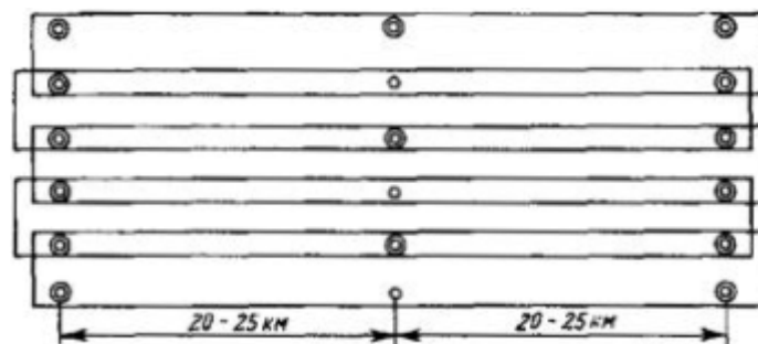
Рис. 7. Съемка в масштабе 1:25000 с сечением рельефа через 5,0 м
