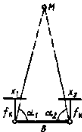
Рис. 38. Схема измерения контрольных направлений
