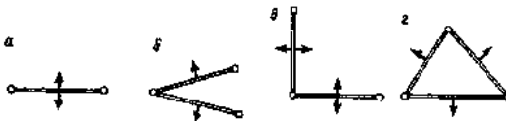
Рис. 36. Схемы расположения базисов фотографирования: а) на узком гребне; б) на широком гребне; в) на разветвленной вершине; г) на округлой вершине
