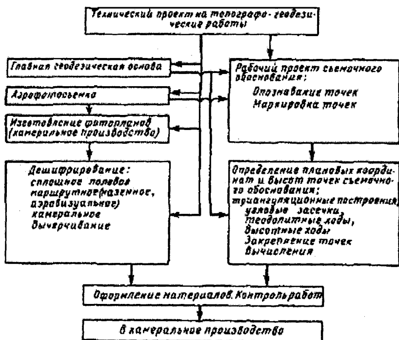
Рис. 1. Технологическая схема полевых работ при стереотопографической съемке
