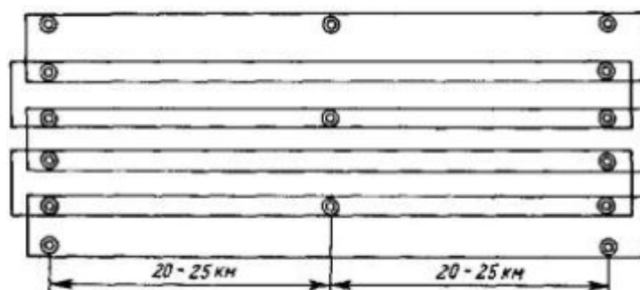
Рис. 8. Съемка в масштабе 1:25000 с сечением рельефа через 10,0 м
